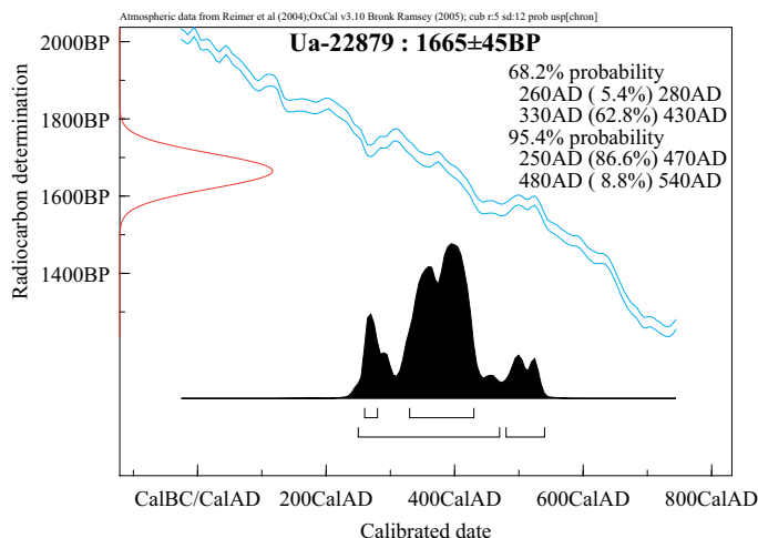
Figur 4. Kalibrerad ^{14}\text{C} -datering av härden.
