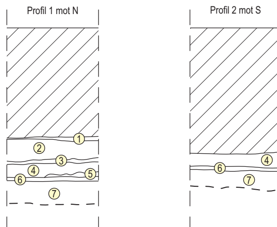
Figur 3. Profilritningar. Skala 1:20.
