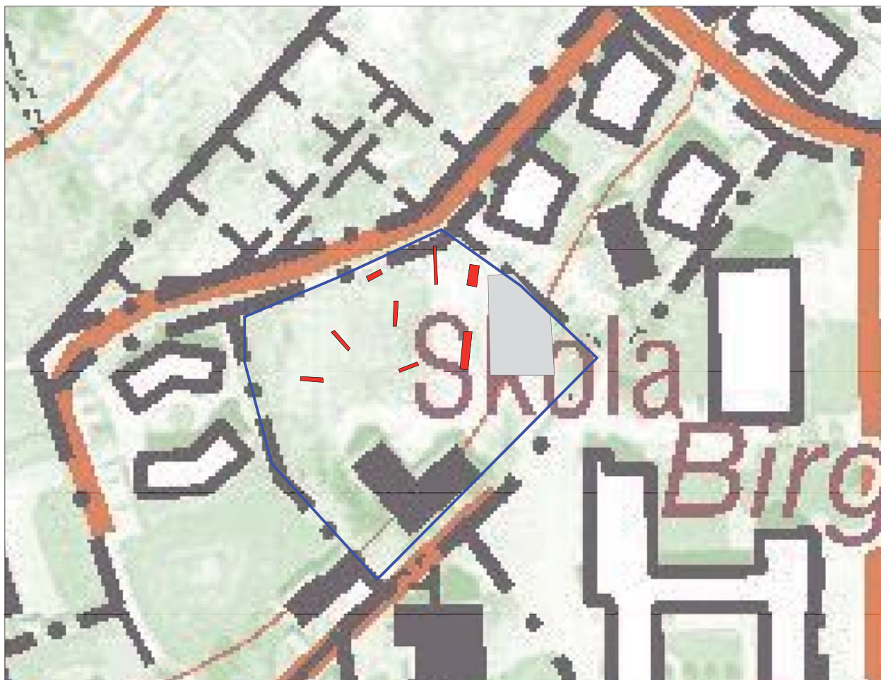
Figur 4. Schaktplan över området. Skala 1:1 500.
