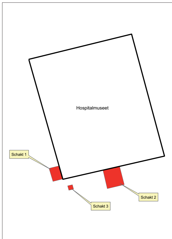
Figur 5. Schaktplan över de tre provgroparna.
