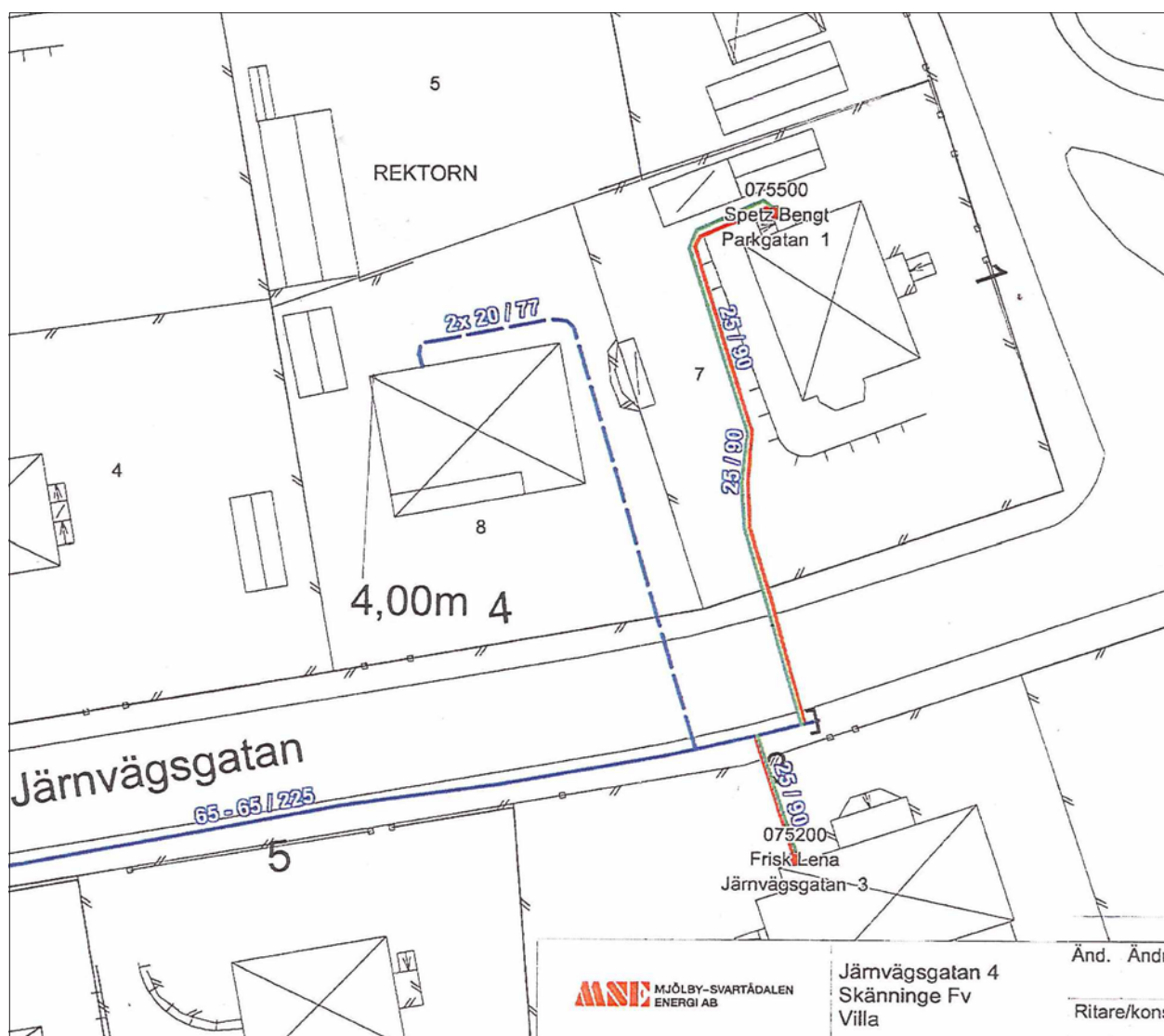
Figur 4. Schaktplan. Den grönda sträckan markerad med blå streckad linje. Karta från uppdragsgivaren MSE. Skala 1:500.
