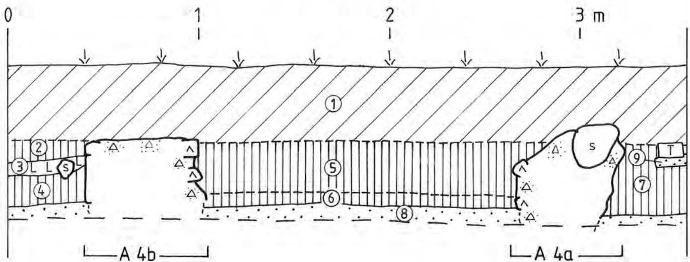
Profil IV mot Ö
